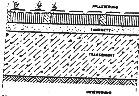
Bild 2: Flächenversickerung durch Setzplattenbau
