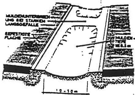
Bild 3: Muldenversickerung
