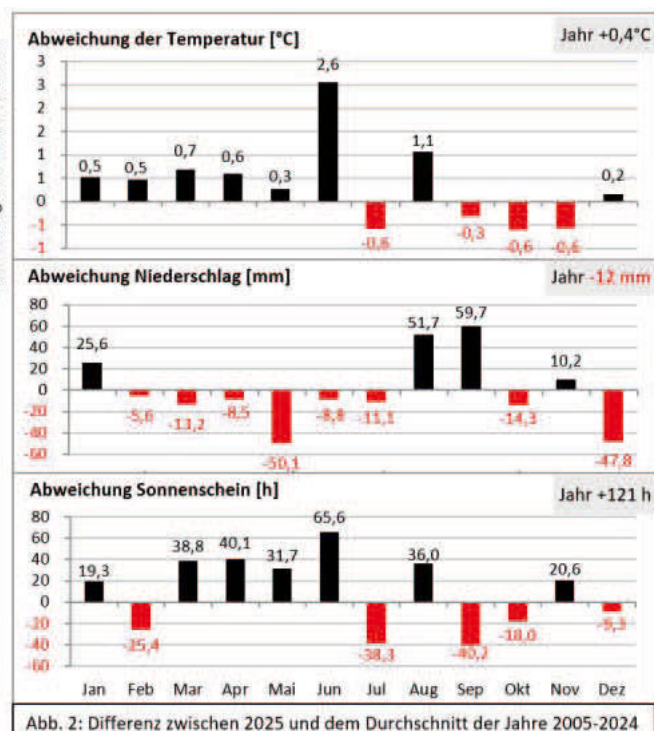
Abb. 2: Differenz zwischen 2025 und dem Durchschnitt der Jahre 2005-2024
