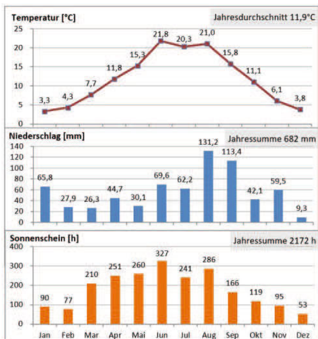
Abb. 1: Monatsdurchschnitte bzw. Monatssummen im Jahr 2025
