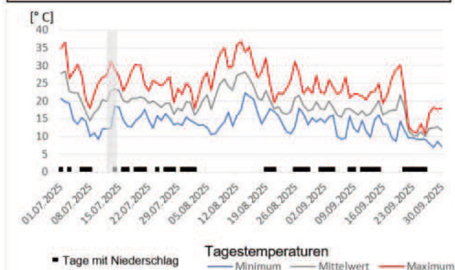
Abb. 3: Temperaturverläufe Juli bis September. Der senkrechte, graue Balken kennzeichnet den Termin des Nepomukfestes.
